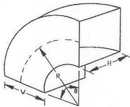
Figura # 2. Codo rectangular de radio suave a 90°.
