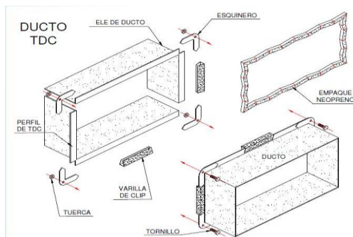
Figura # 8. Elementos de la conexión TDC
