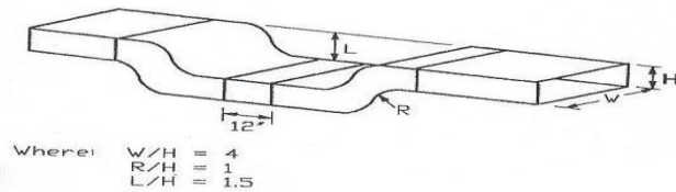
Figura # 3. Ducto rectangular para evitar obstrucciones.
